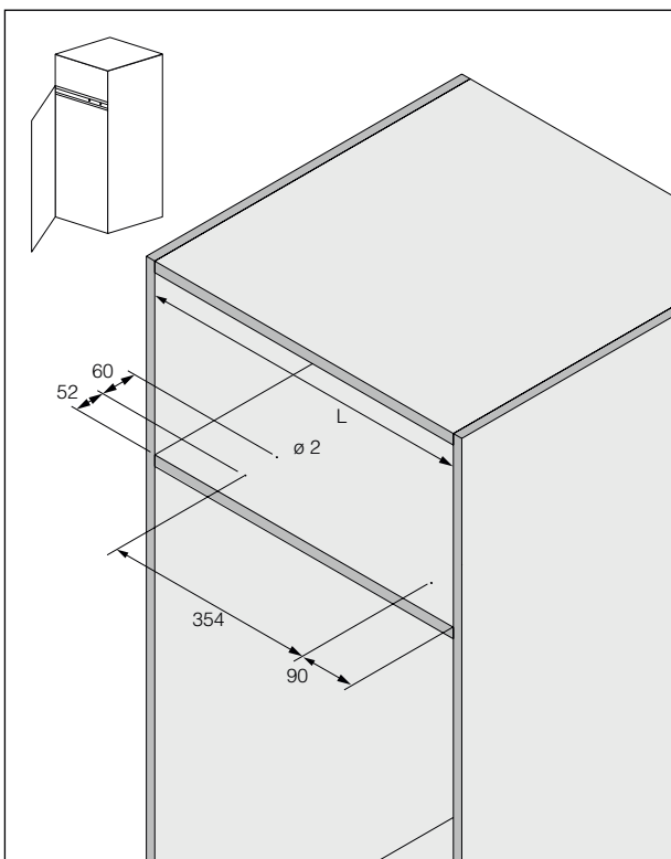
Taladros puerta de frigorífico con sujeción a la izquierda
